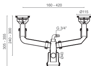
DUPLO C/ VÁLVULAS CESTO DOBLE CON VÁLVULA DE CESTILLA DUAL WITH VALVE BASKET DOUBLE AVEC VIDAGE À PANIER
