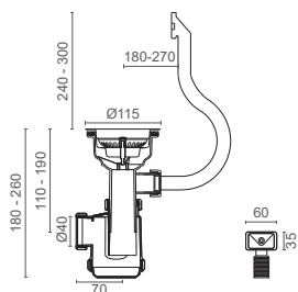
SIMPLES C/ VÁLVULA CESTO E AVISADOR SIMPLE CON VÁLVULA DE CESTILLA Y REBOSADERO SIMPLE WITH VALVE BASKET AND OVERFLOW SIMPLE AVEC VIDAGE PANIER ET TROP-PLEIN
