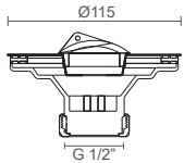
VÁLVULA SIMPLES VALVULA SIMPLE | SIMPLE VALVE | VIDAGE SIMPLE
