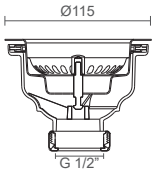
VÁLVULA C/ CESTO INOX VALVULA DE CESTILLA | VALVE BASKET | VIDAGE PANIER
